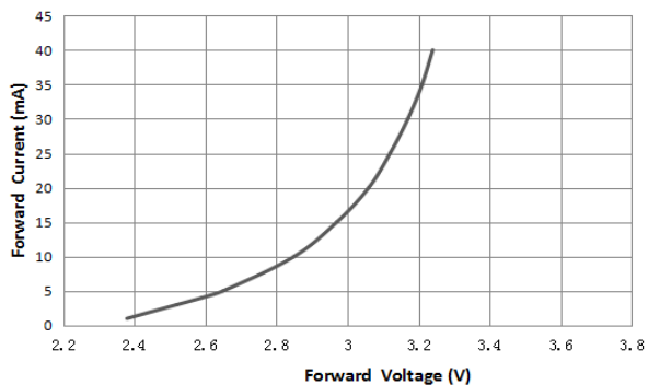
伏安特性曲线
