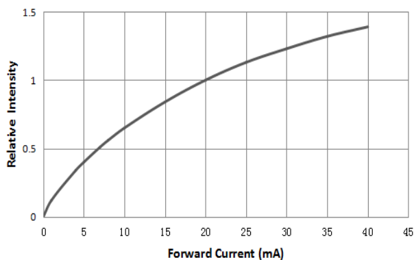
相对光强与电流特性曲线
