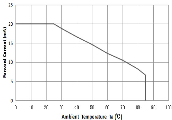
最大正向电流与环境温度特性曲线
