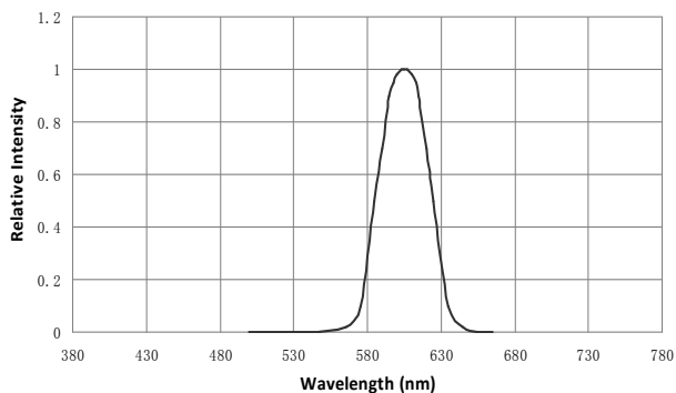
光谱分布特性曲线
