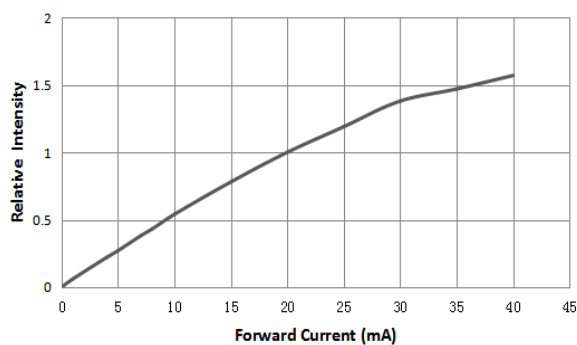
相对光强与电流特性曲线
