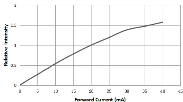
相对光强与电流特性曲线
