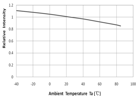
相对光强与环境温度特性曲线
