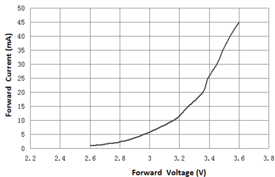
伏安特性曲线
