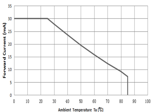
最大正向电流与环境温度特性曲线
