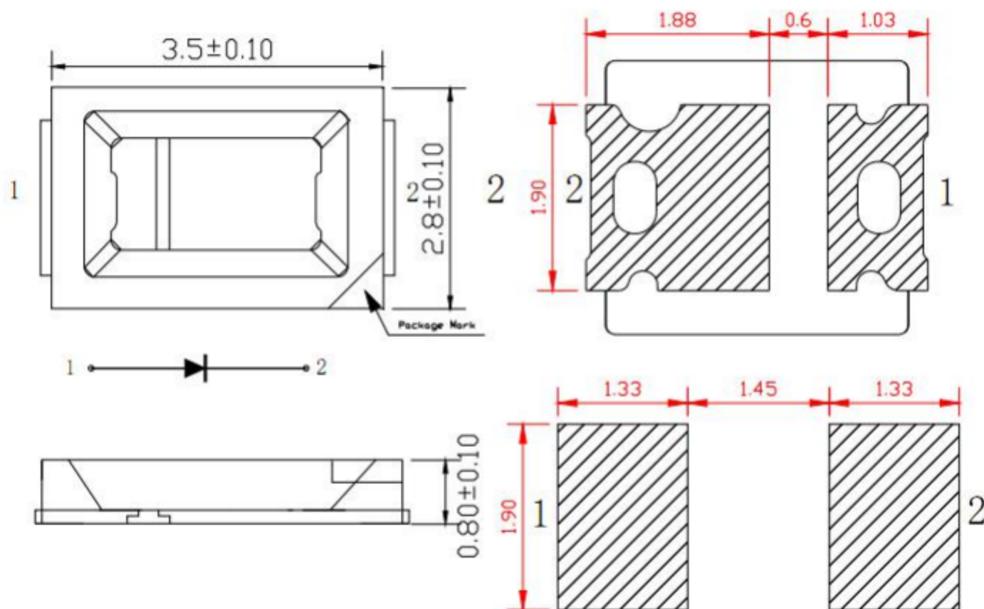
焊盘图
