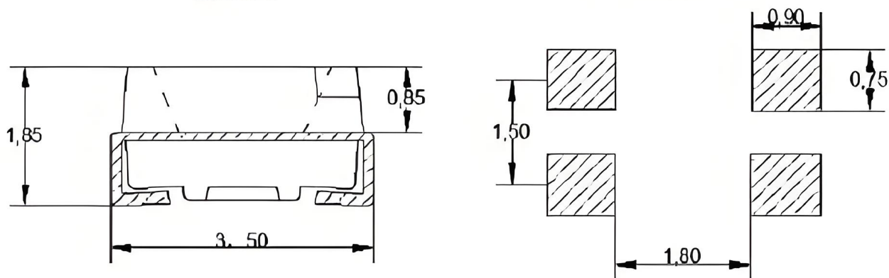
侧面图
