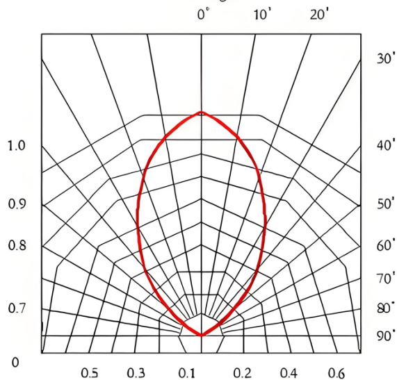
相对辐射程度与空间角度关系
