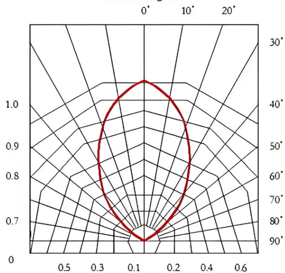
相对辐射强度与空间角度关系
