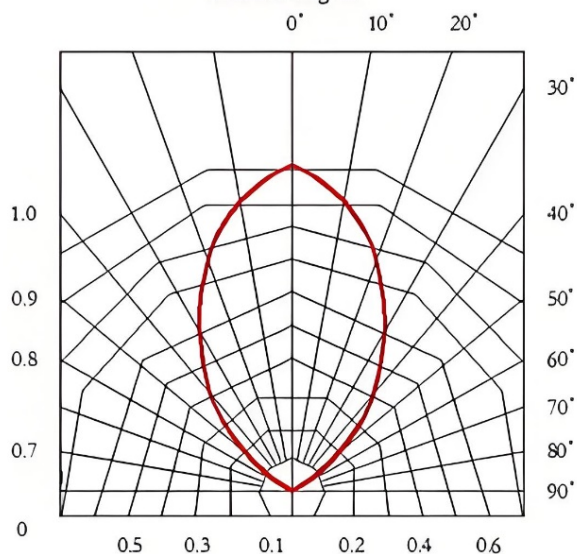
相对辐射强度与空间角度关系
