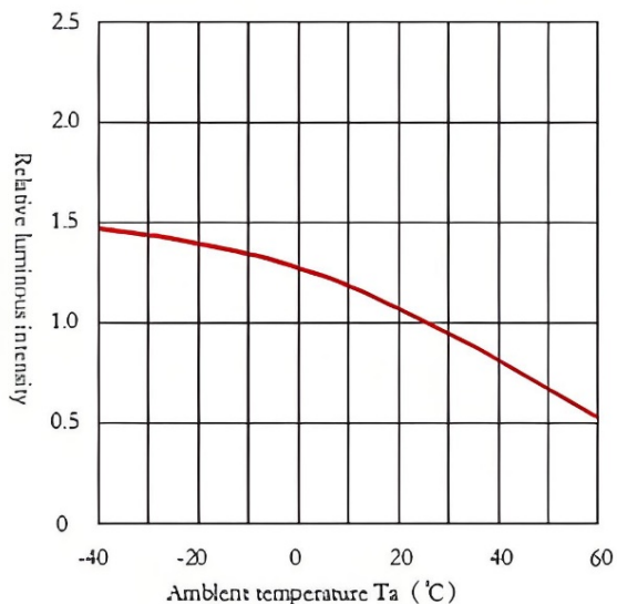
环境温度与相对光强的关系
