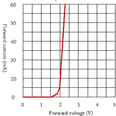
正向电压与正向电流的关系
