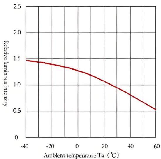
环境温度与相对光强的关系
