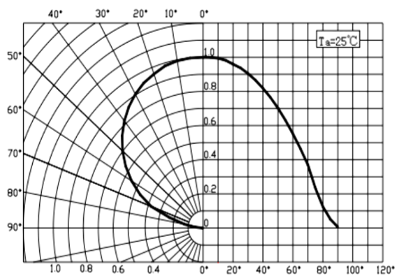
辐射特性曲线
