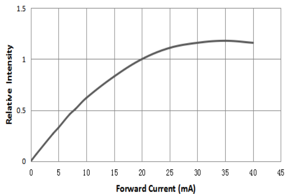
相对光强与电流特性曲线
