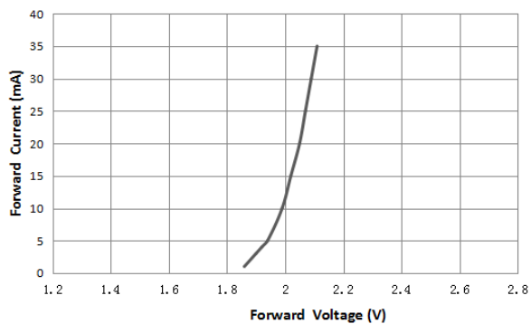
伏安特性曲线
