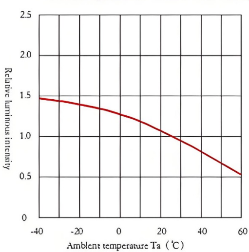
环境温度与相对光强的关系
